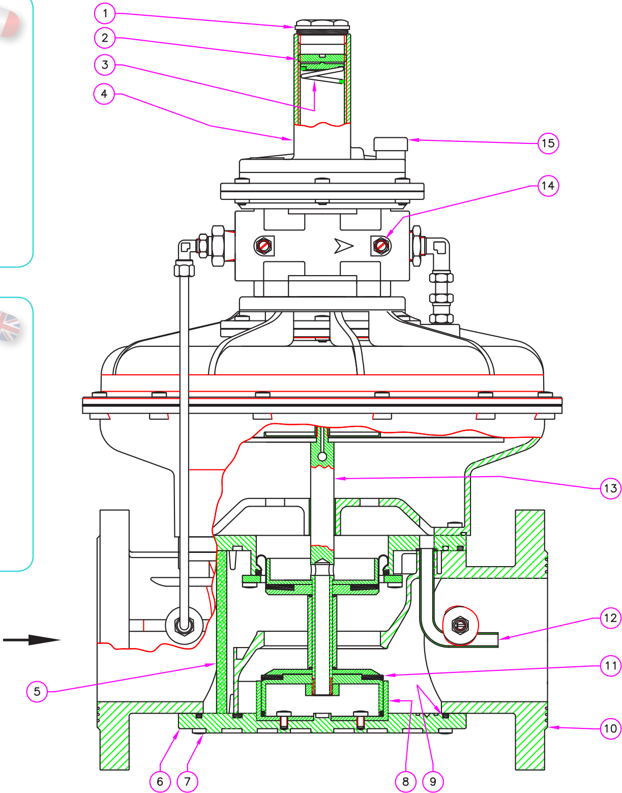
fig. 4: DN 65 - DN 80 - DN 100 P2 = 200÷450 mbar
