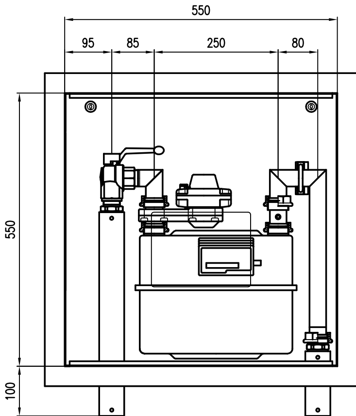
PE D32 SDR11
