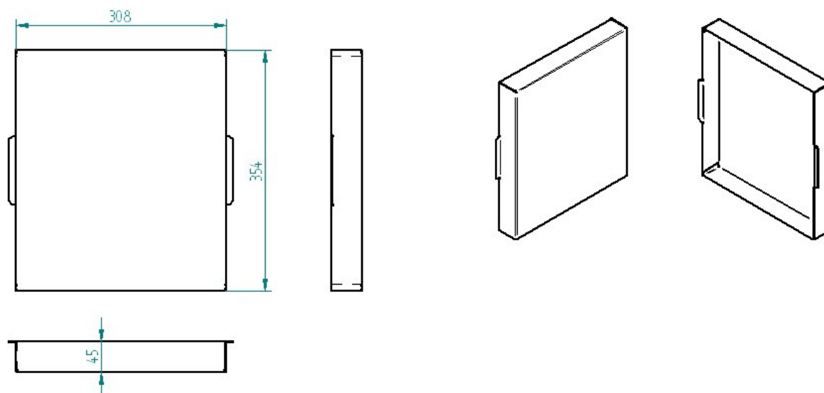
2. ábra előlap nézeti rajzok
