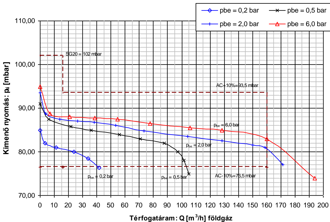
VF-160 / 76 szabályozó jelleggörbe - 85 mbar
